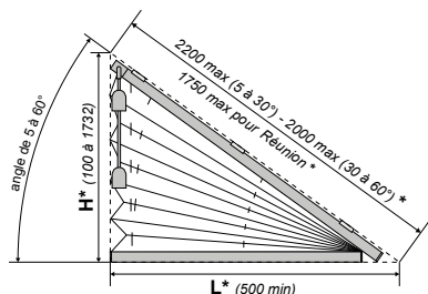
Triangle manœuvrable
