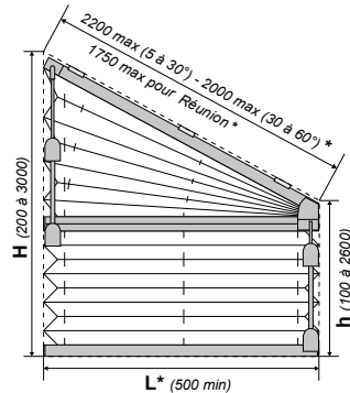
Trapèze manœuvrable
