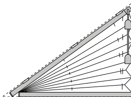
Triangle manœuvrable
