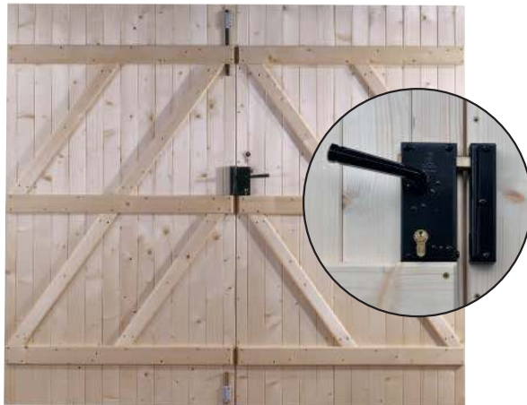
2 vantaux Sapin du Nord : serrure 1 point, verrou baïonnette, sur gond à sceller
