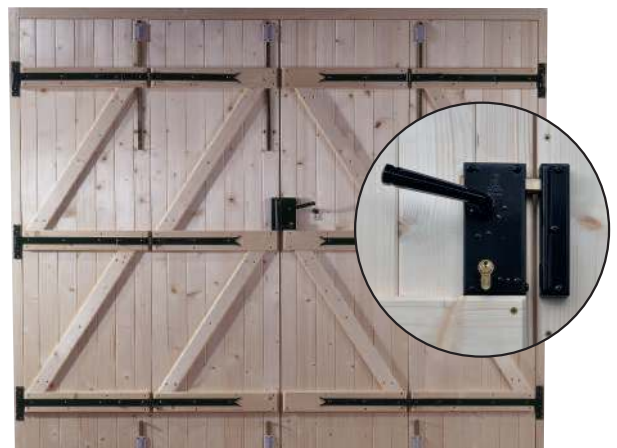
4 vantaux repliables Sapin du Nord : serrure 1 point, verrou baïonnette, bâti de 65 x 55 mm, avec bâti cintré dessous sans seuil
